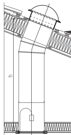
конструкция SFP
