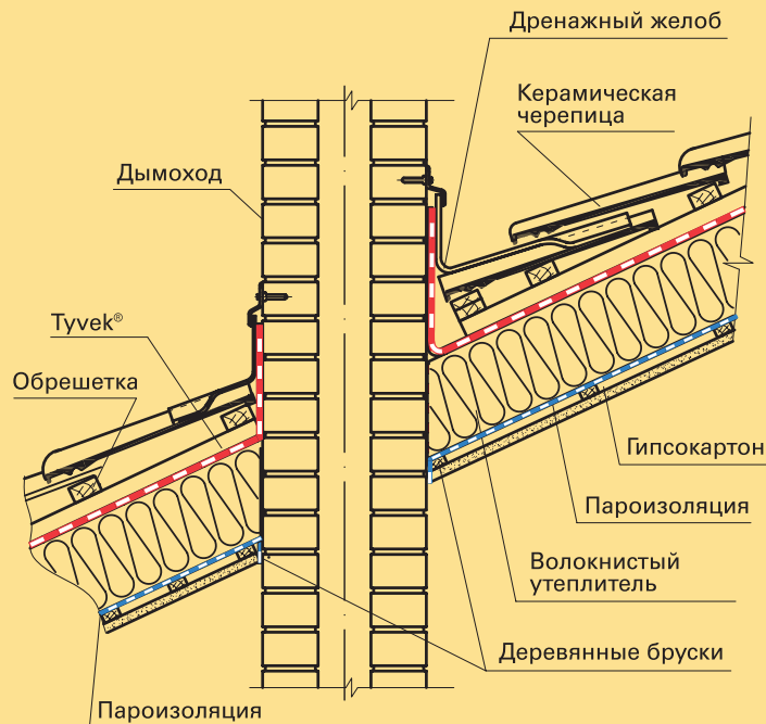
Рис. 3 Дымоход
