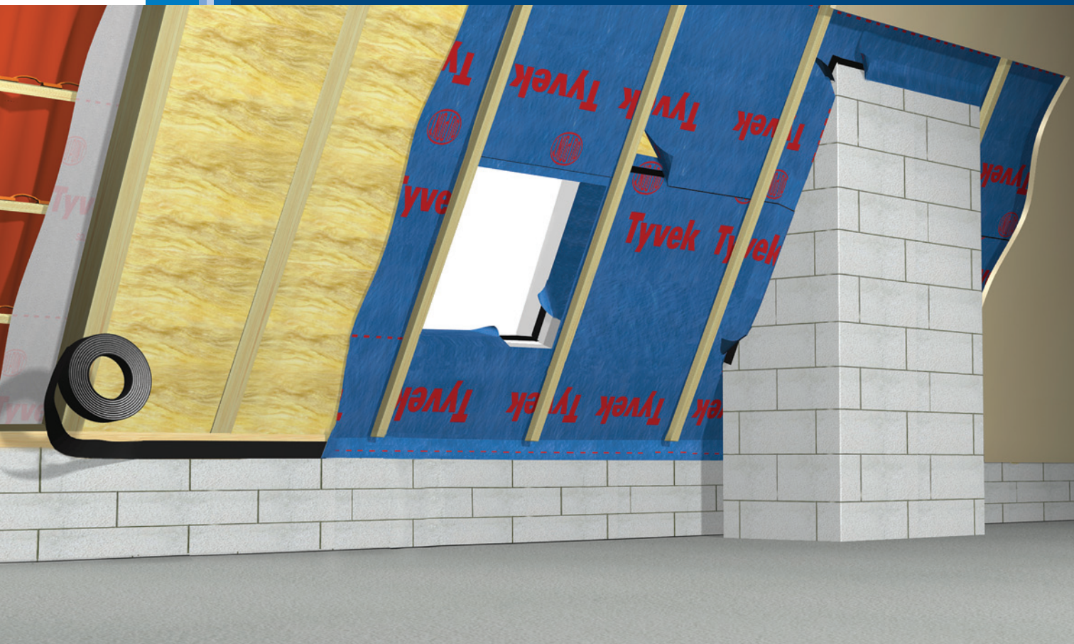
Рис. 10 Монтаж пароизоляции
