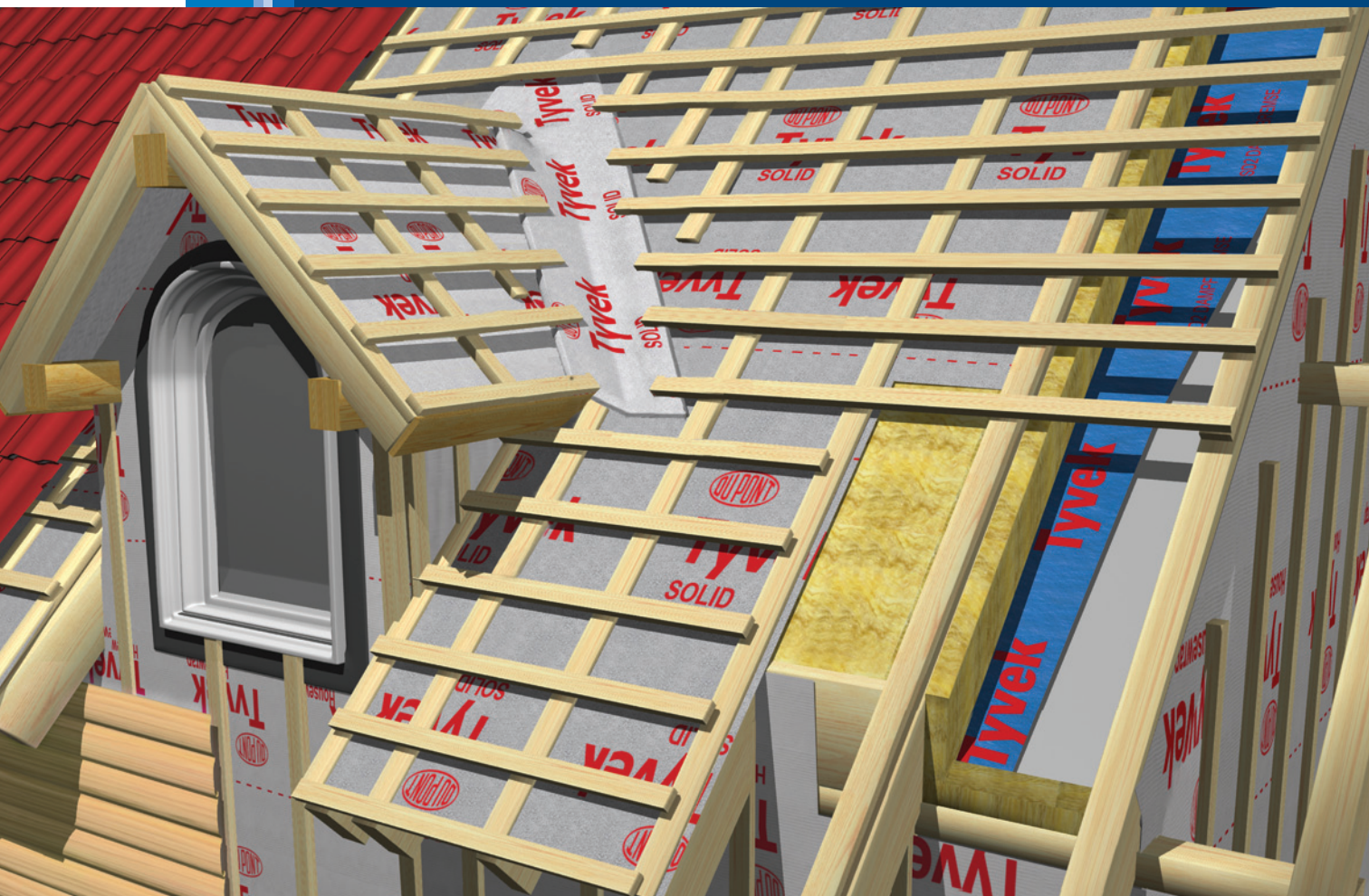
Рис. 1 Устройство утепленной мансарды
