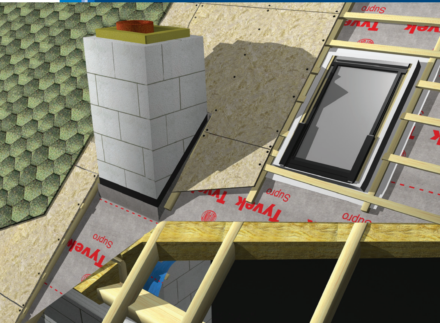
Рис. 4 Дымоход и мансардное окно
